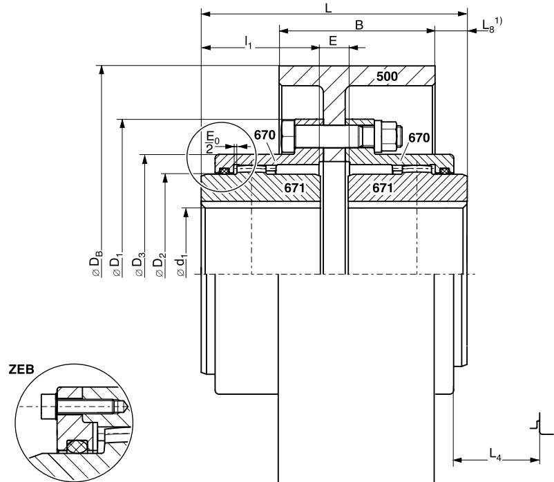
ZEA mit integriertem O-Ring, ZEB mit separatem O-Ring-Deckel ZEA with integrated O-ring, ZEB with separate o-ring cover ZEA avec joint torique intégré, ZEB avec couvercle du joint torique séparé
